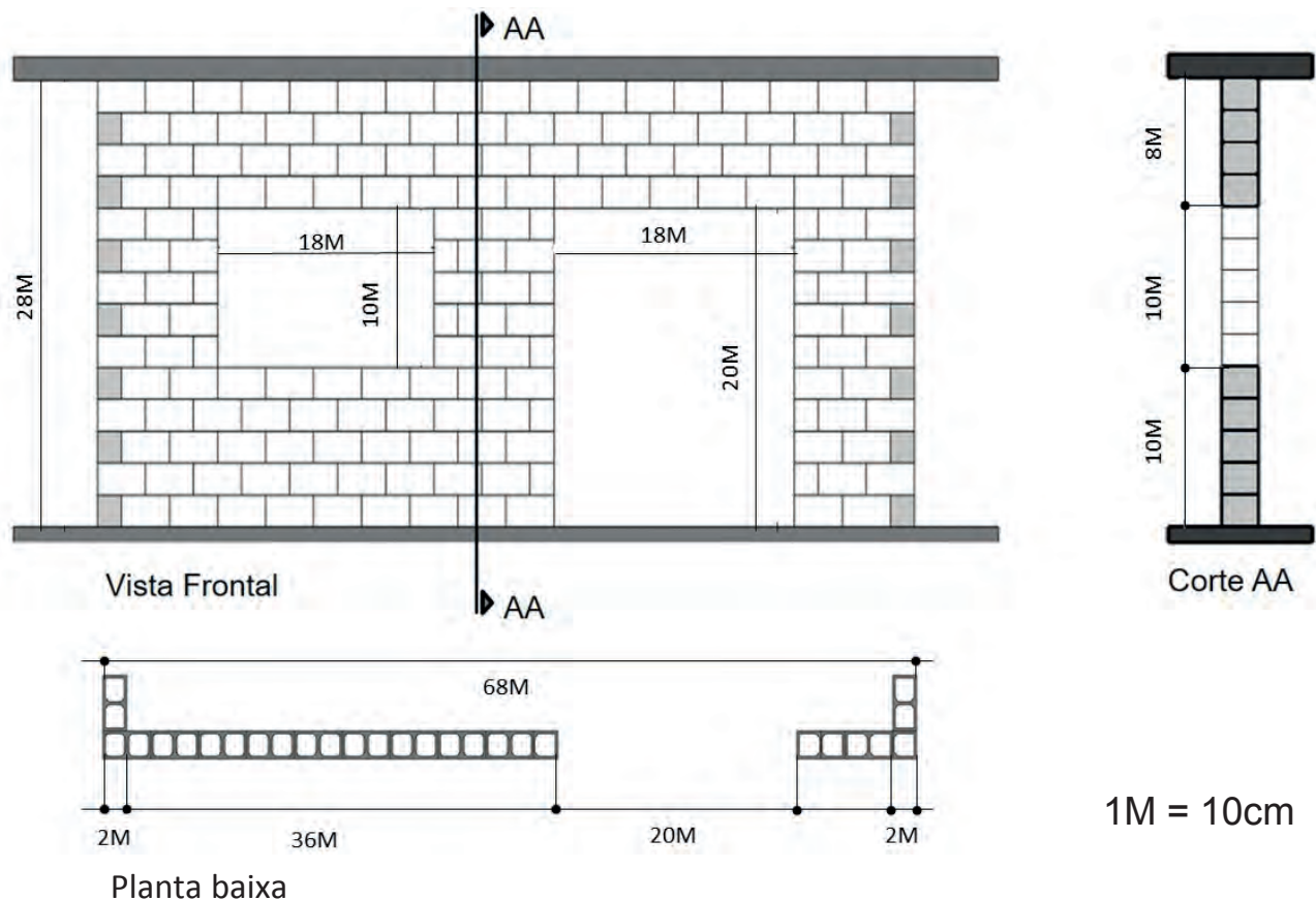
Figura 41. Representação de trechos de projeto com coordenação modular.
