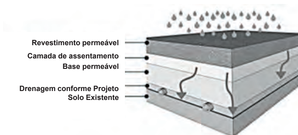
Figura 62. Representação gráfica de pavimentos permeáveis.
